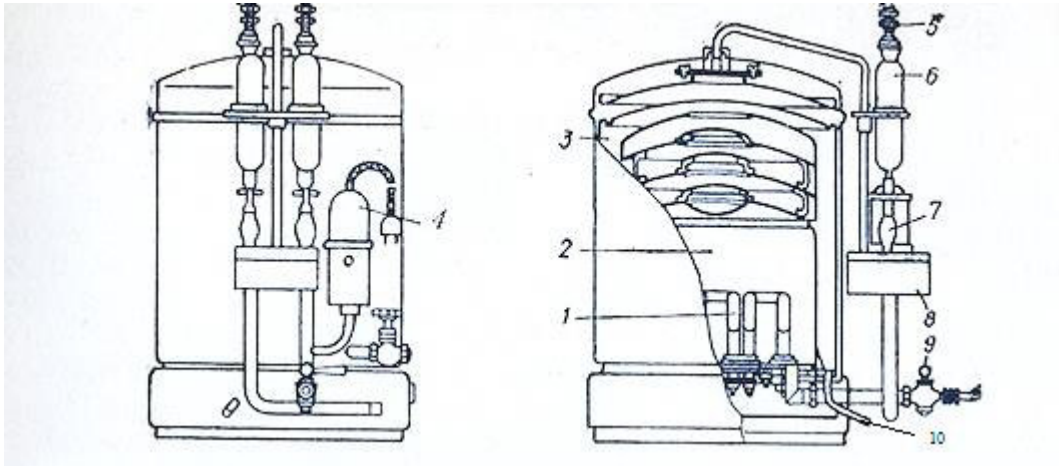
Рис. 1. Аквадистиллятор А-10 для получения воды для инъекций
